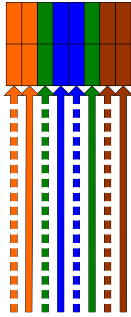
Data TIA/EIA 568B
